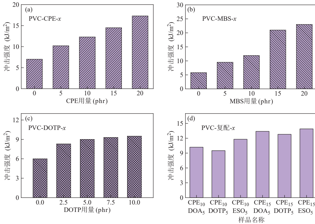
图6 增韧剂与增塑剂对PVC耐折板皮层实验样品冲击性能的影响：(a) CPE、(b) MBS和(c) DOTP用量的影响；(d) CPE与增塑剂复配的影响
