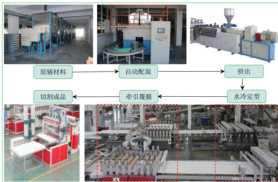
图4 PVC耐折板的生产流程
